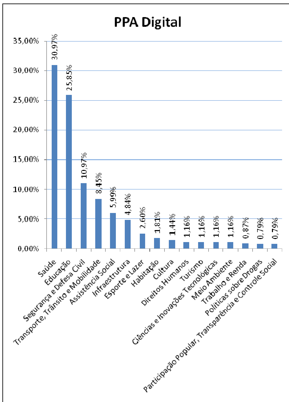
Gráfico 31 - PPA Digital
